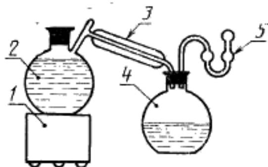
1 — электроплитка; 2 — дистилляционная колба; 3 — холодильник; 4 — колба-приемника; 5 — предохранительная воронка
