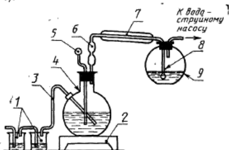
1 — промытые сосуды, заполненные серной кислотой и водой; 2 — электролитка; 3 — стеклянная трубка диаметром 6—7 мм; 4 — реакционная колба из термостойкого стекла вместимостью 300 см 3 ; 5 — капельная воронка с краном; 6 — дефлегматор; 7 — холодильник; 8 — барботер; 9 — сосуд для поглощения аммиака
